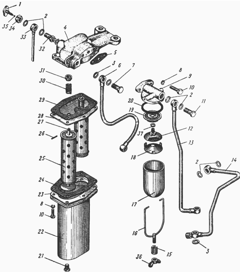
Рис. 24. Фильтр грубой очистки топлива. Фильтр тонкой очистки топлива
